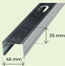
Montante Pladur® M 48/35 Z1
