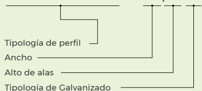
Montante Pladur® M 48/35 Z1
