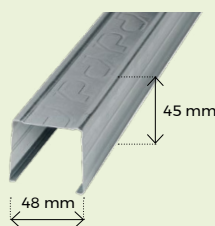
Montante Pladur® M 48/45 XL Z1
