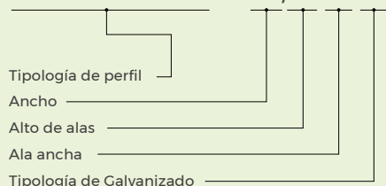
Montante Pladur® M 48/45 XL Z1
